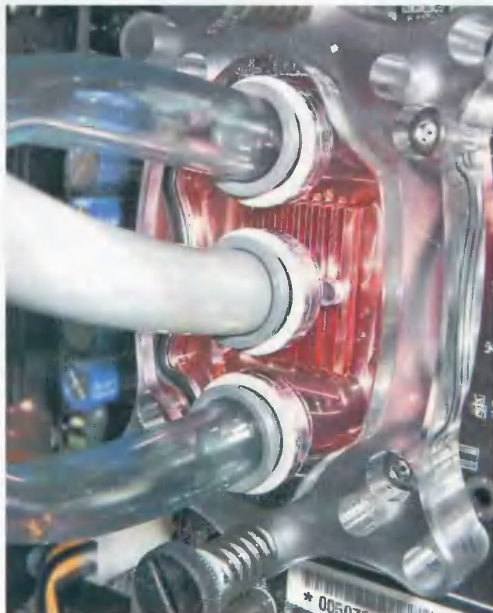
Примерно так выглядит двухпоточный ватерблок с тремя патрубками. Как видите, красивая и эффективная конструкция.
