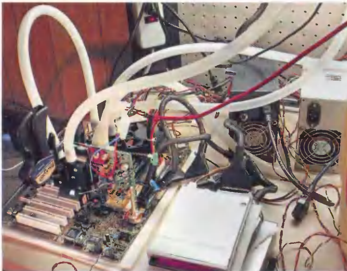
Присутствие элемента Пельтье выдают лишь два толстых проводка под ватер-блоком и второй блок питания.
