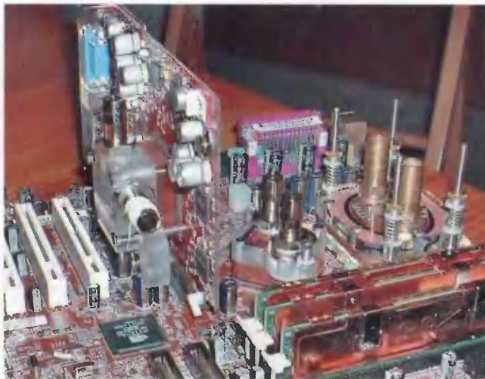
Ватерблоки с прозрачными крышками стали очень популярны благодаря приятному внешнему виду и относительной простоте конструкции.
